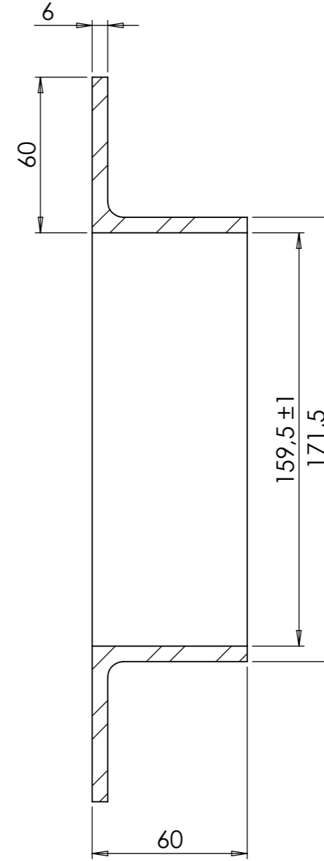
SECTION A-A
