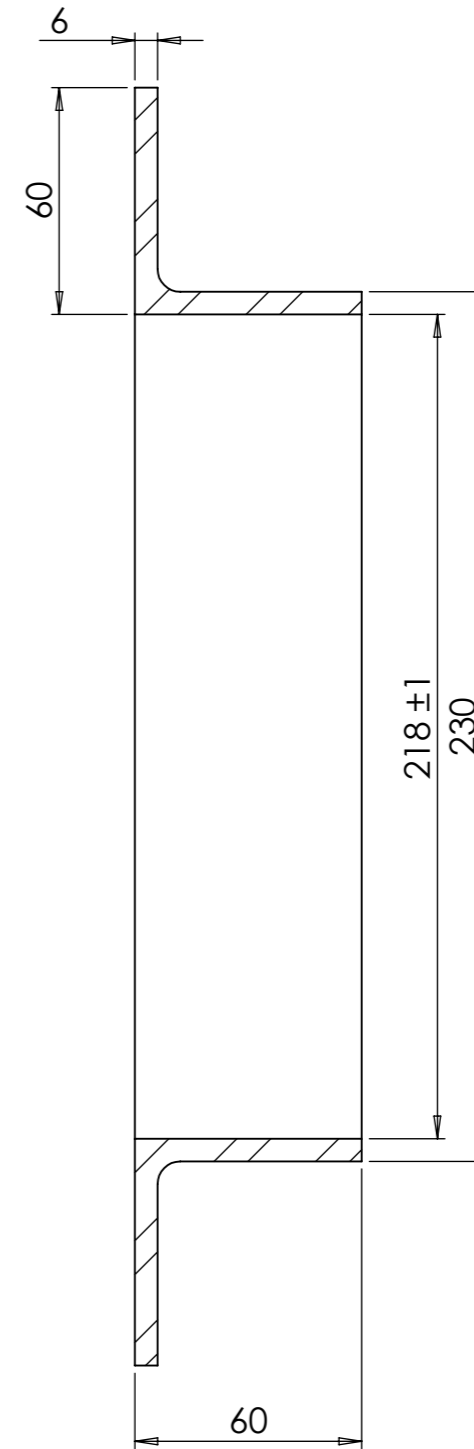
SECTION A-A
