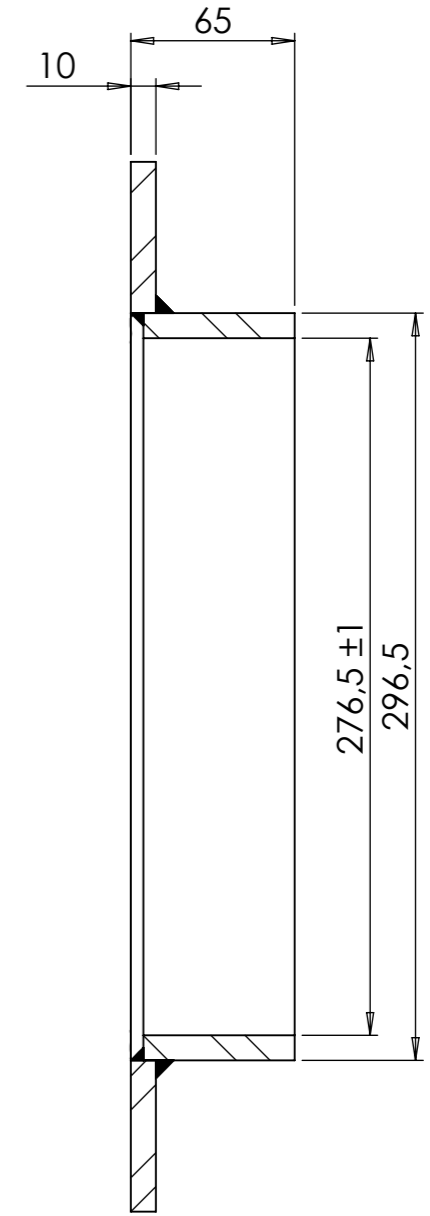
SECTION A-A
