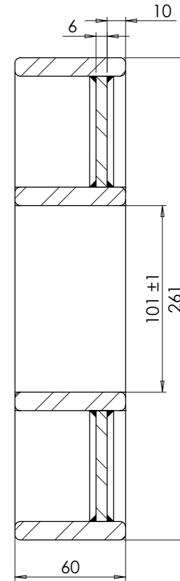
SECTION A-A
