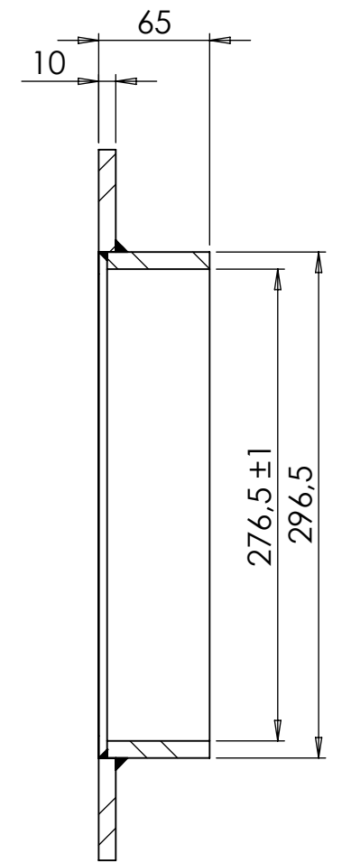
SECTION A-A
