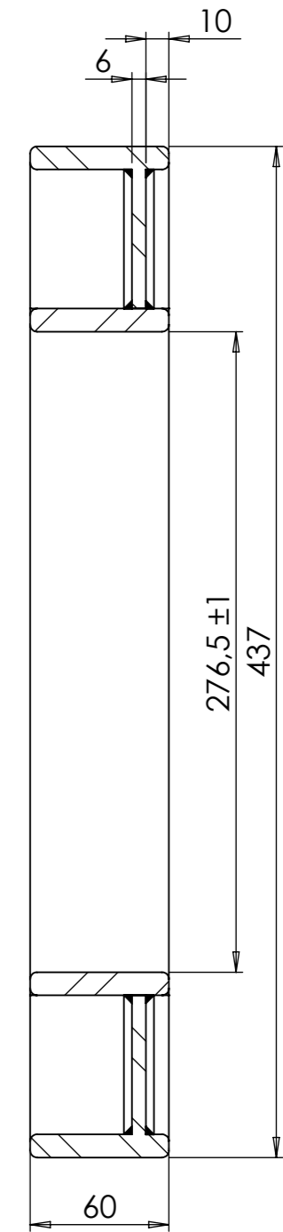
SECTION A-A
