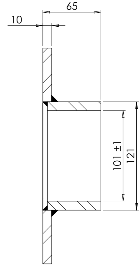
SECTION A-A
