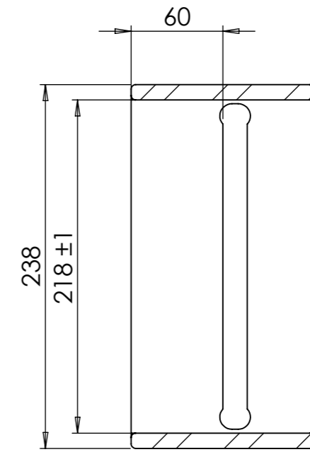
SECTION A-A
