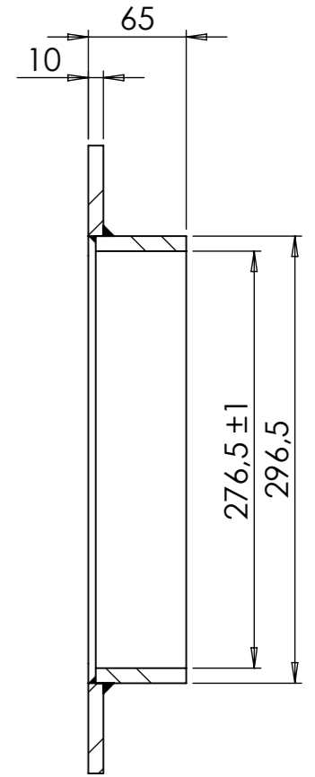
SECTION A-A
