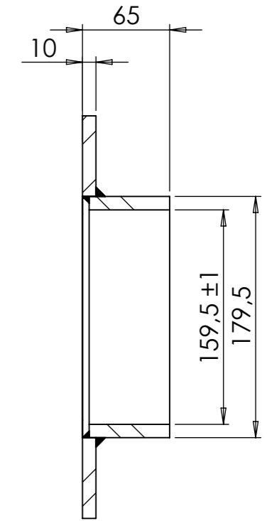
SECTION A-A
