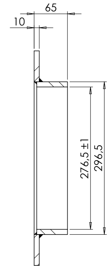
SECTION A-A
