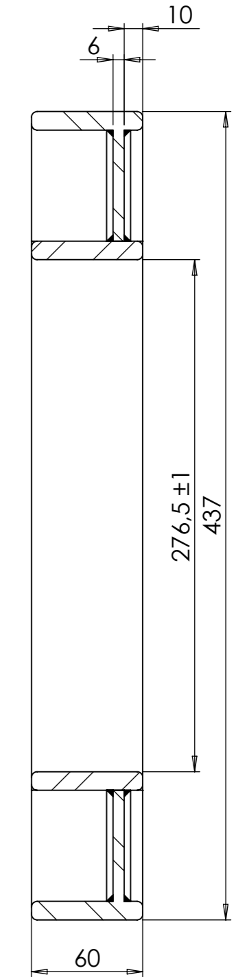
SECTION A-A
