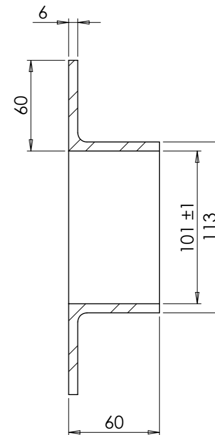
SECTION A-A
