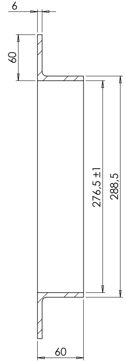
SECTION A-A
