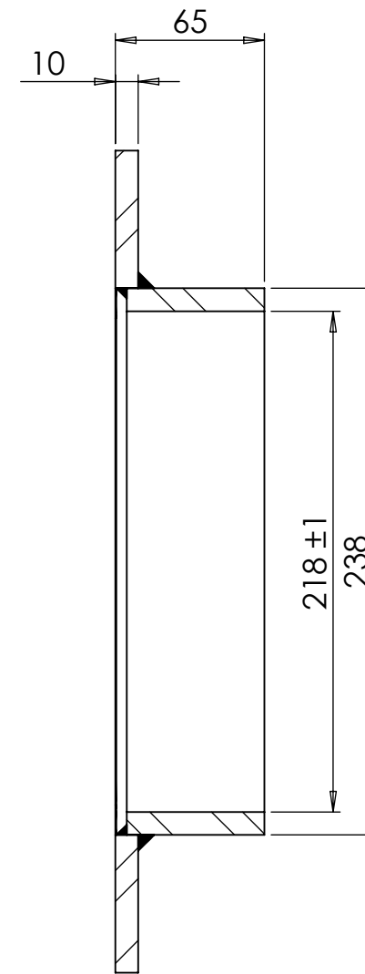
SECTION A-A
