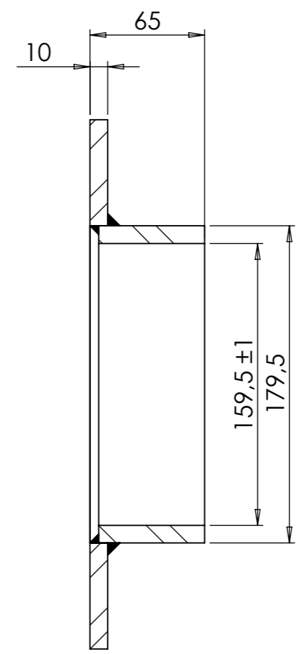
SECTION A-A
