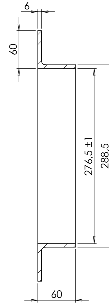
SECTION A-A
