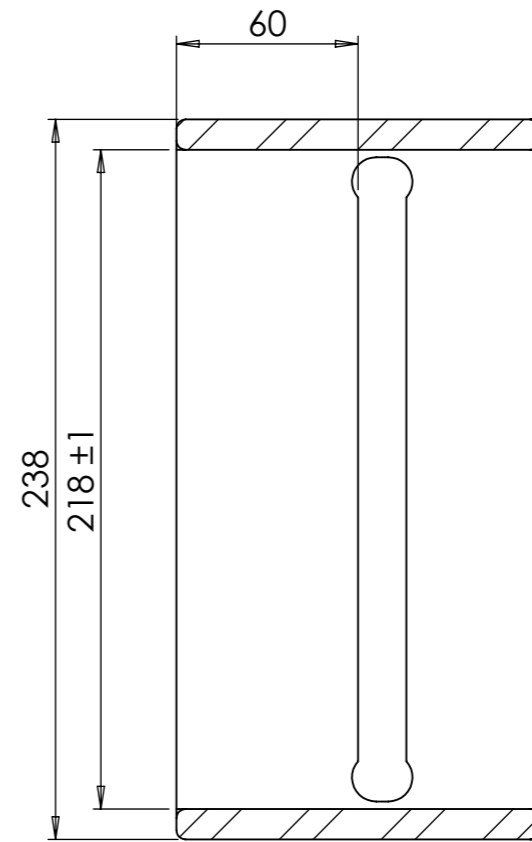
SECTION A-A
