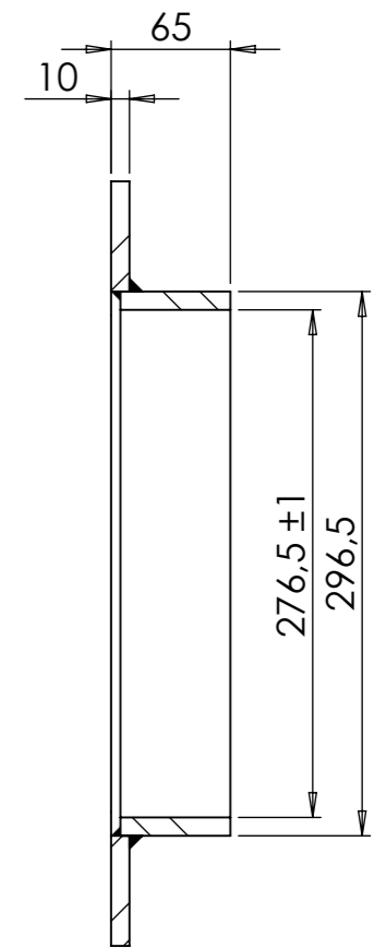
SECTION A-A
